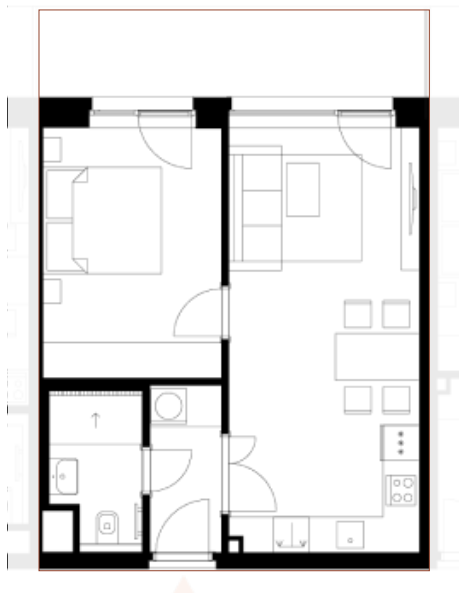
DISPOZICE — VÝŘEZ Z PODLAŽNÍ KRESBY
